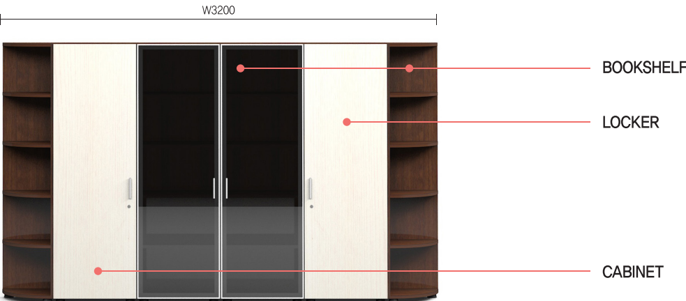
TOCN400R + TOCB064(L) + TOBS064G(L) + TOBS064G(R) + TOLK064(R) + TOCN400R 최우 대칭 구조로 안정적이며 중앙의 유리 도어가 W1200mm로 넓게 설치되어 시각적인 답답함을 감소하여 줍니다.
